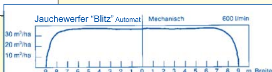
Streubild des Jauchewerfers Blitz AH
