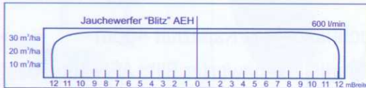
Streubild des Jauchewerfers Blitz AEH
