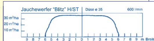
Streubild des Streutellers bei 600l/min
